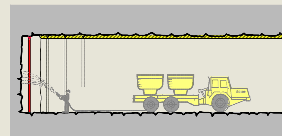
Bogen setzen Spritzbeton aufbringen
