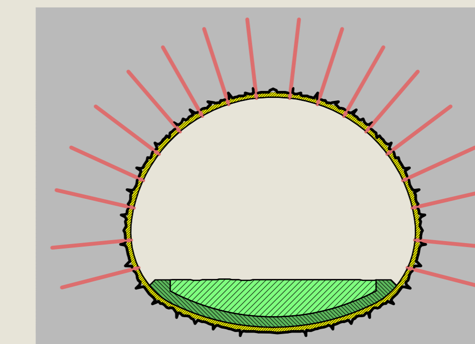
Sohlgewölbe / Sohlfüllbeton einbauen
