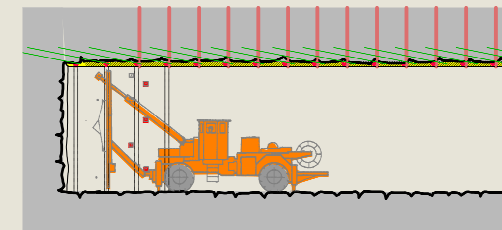
Spieße bohren und Anker setzen
