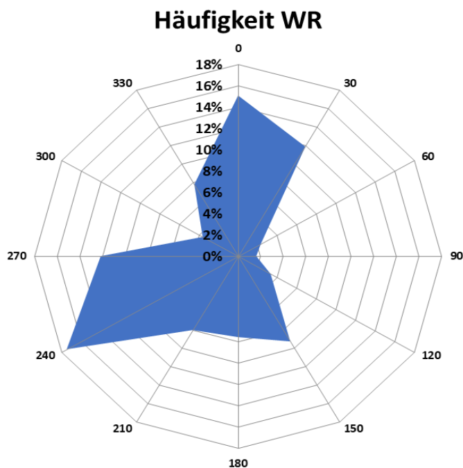
Abbildung 9 Windrichtungsverteilung im Monat September 2022 (nur HMW mit Windgeschwindigkeiten > 0,5 m/s)
