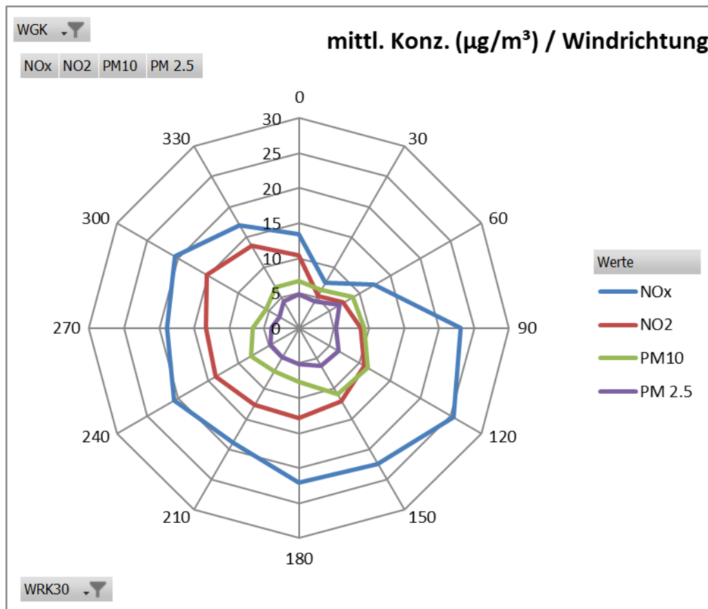
Abbildung 11 Windrichtungsabhängigkeit der Immissionsbelastung im Monat September 2022 (es sind nur Datensätze mit Windgeschwindigkeiten > 0,5 m/s in der Darstellung berücksichtigt)
