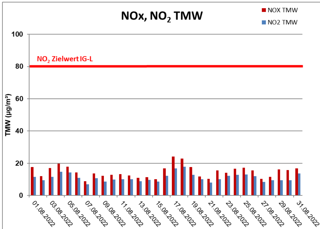
Abbildung 4 Zeitlicher Verlauf der NO 2 - und NO x -Tagesmittelwerte an der Beweissicherungsmessstelle Angath
