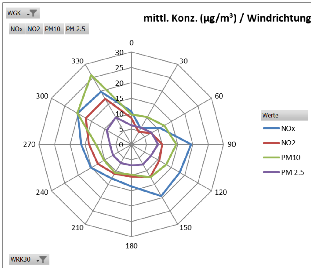
Abbildung 11 Windrichtungsabhängigkeit der Immissionsbelastung im Monat August 2022 (es sind nur Datensätze mit Windgeschwindigkeiten > 0,5 m/s in der Darstellung berücksichtigt)
