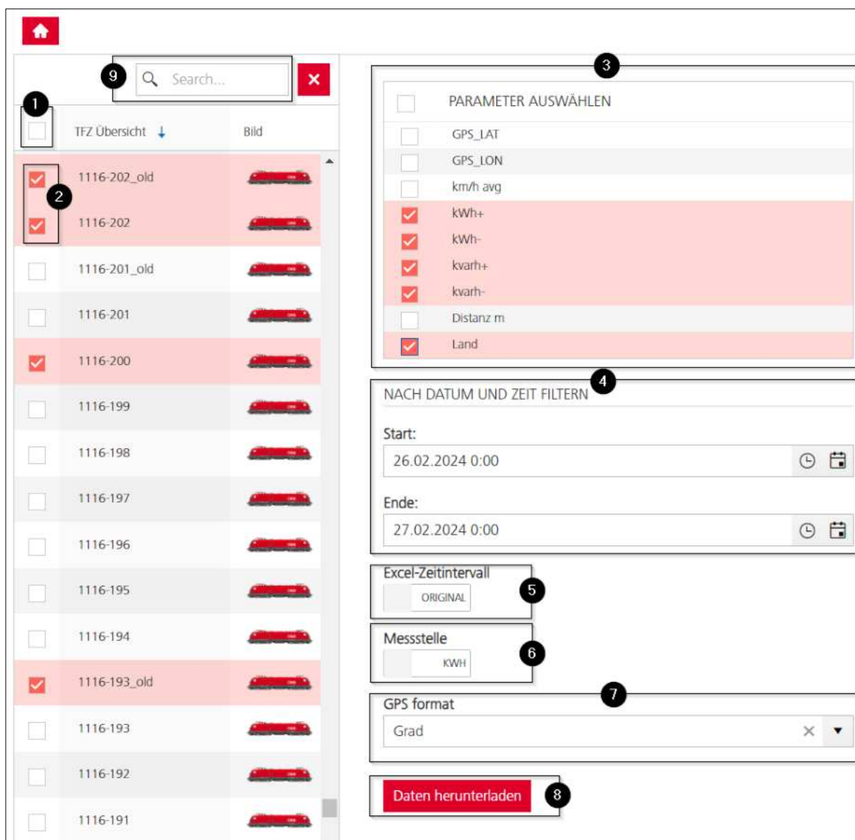
Abbildung 28 – Datenexport Einstellungen
