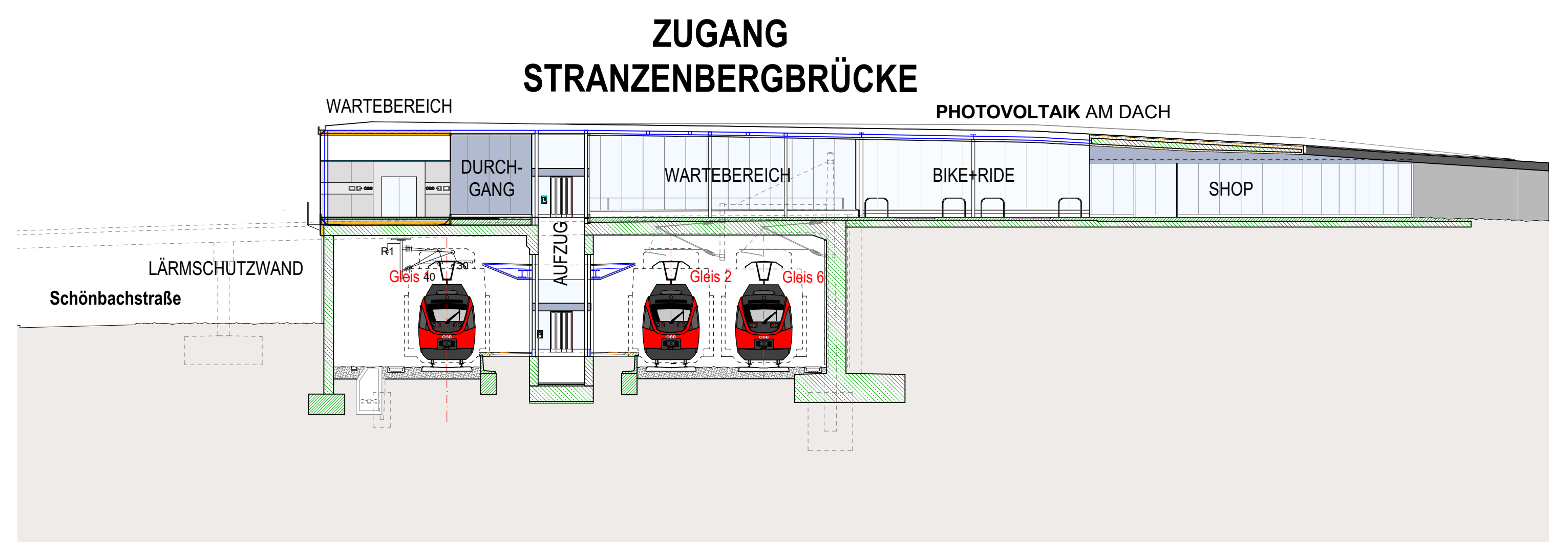
SCHNITT 1-1
