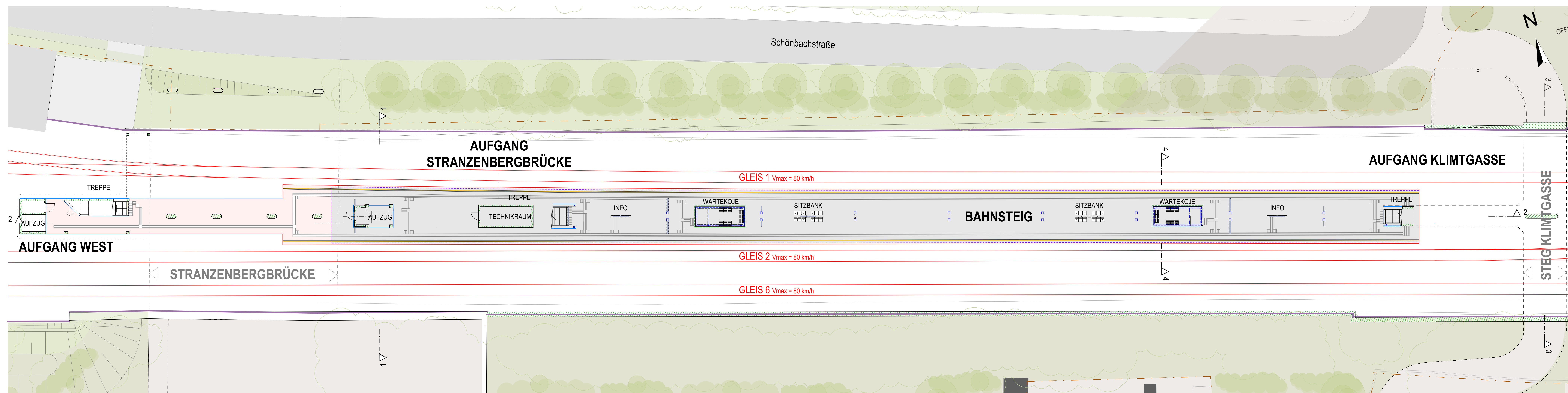
BAHNSTEIGEBENE
