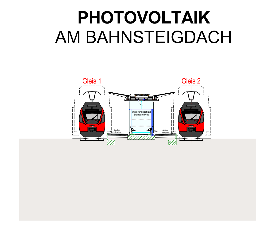
SCHNITT 4-4
