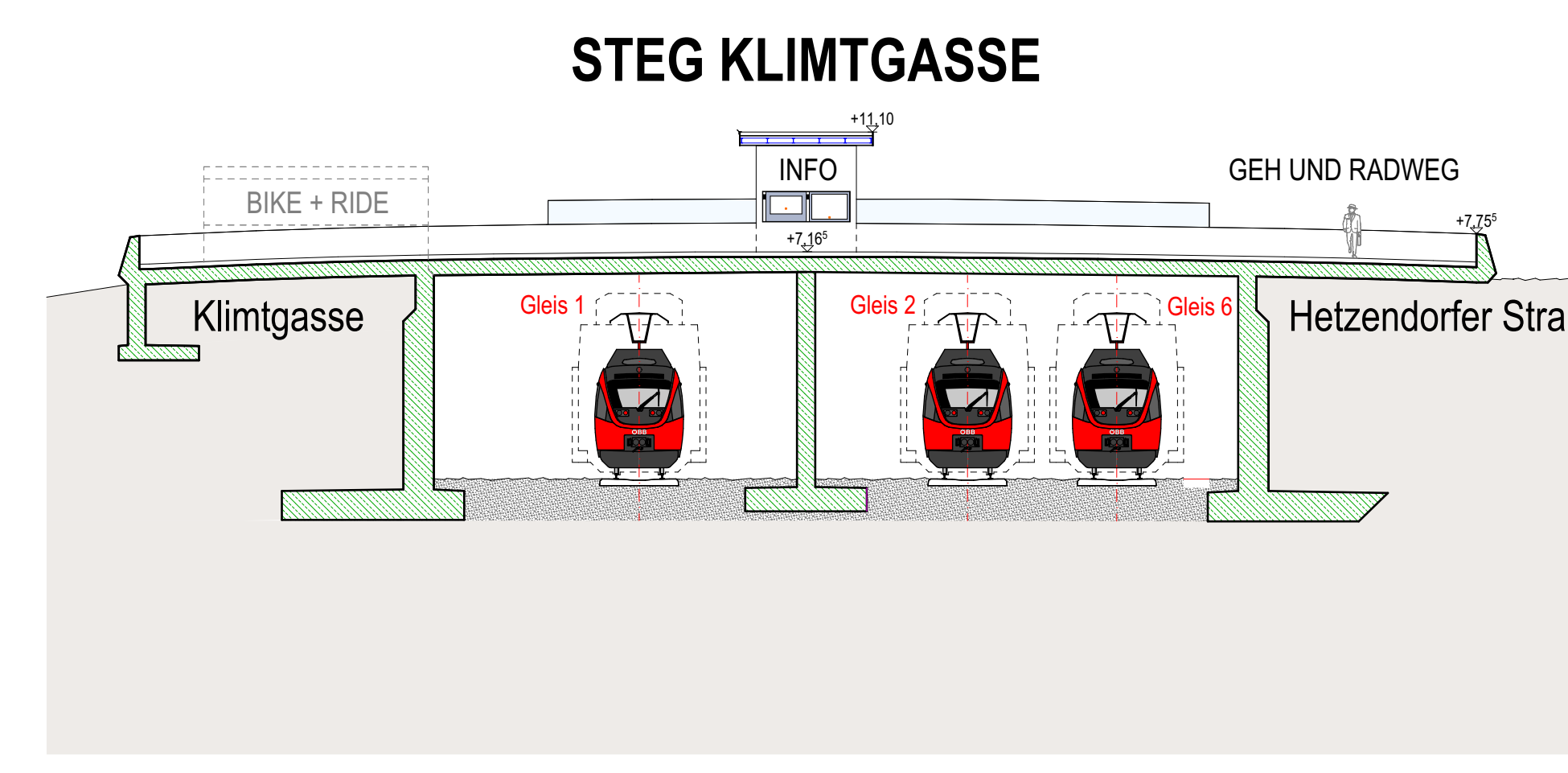
SCHNITT 3-3
