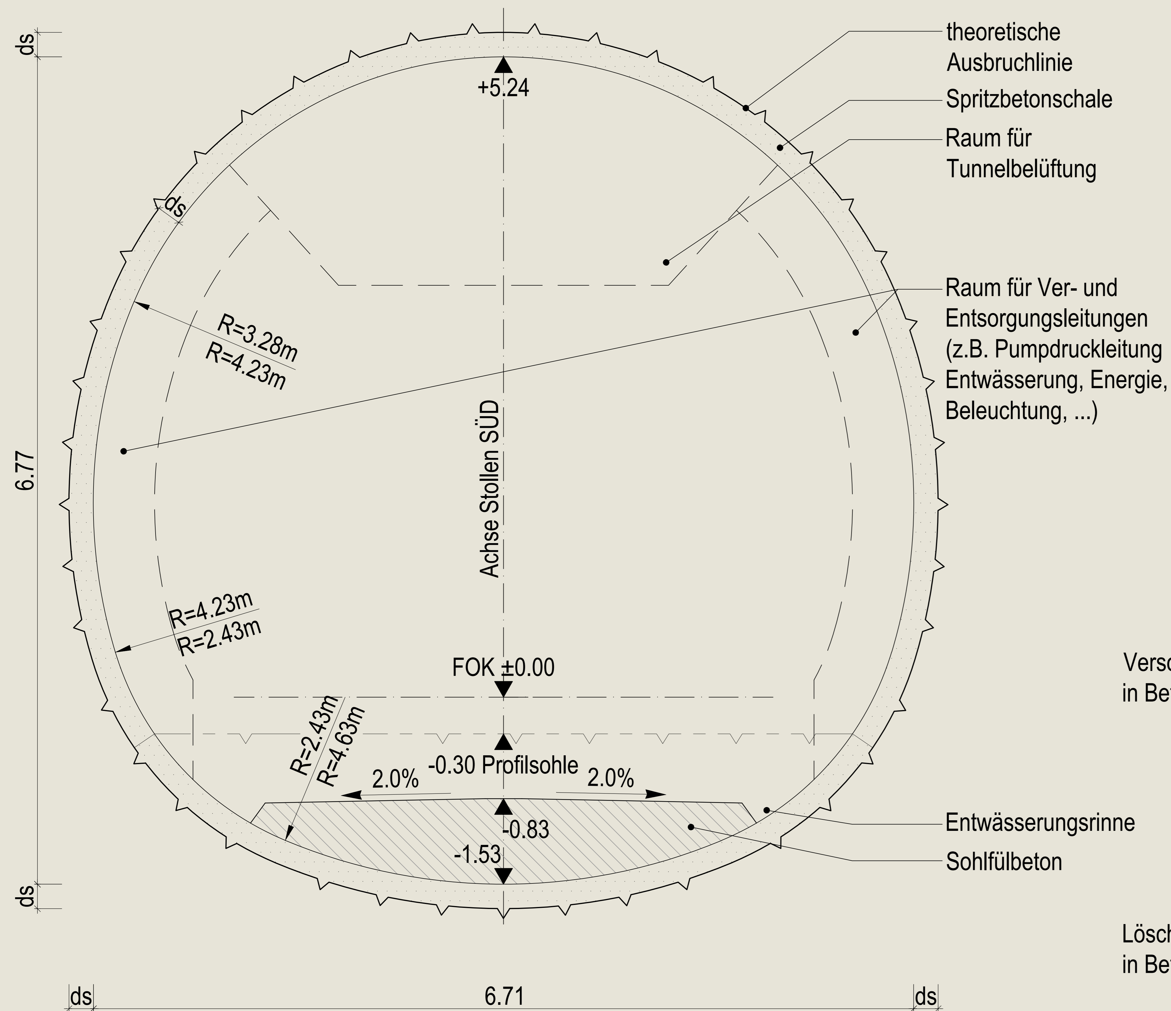
Rohbaustollen Angath ohne Innenschale
