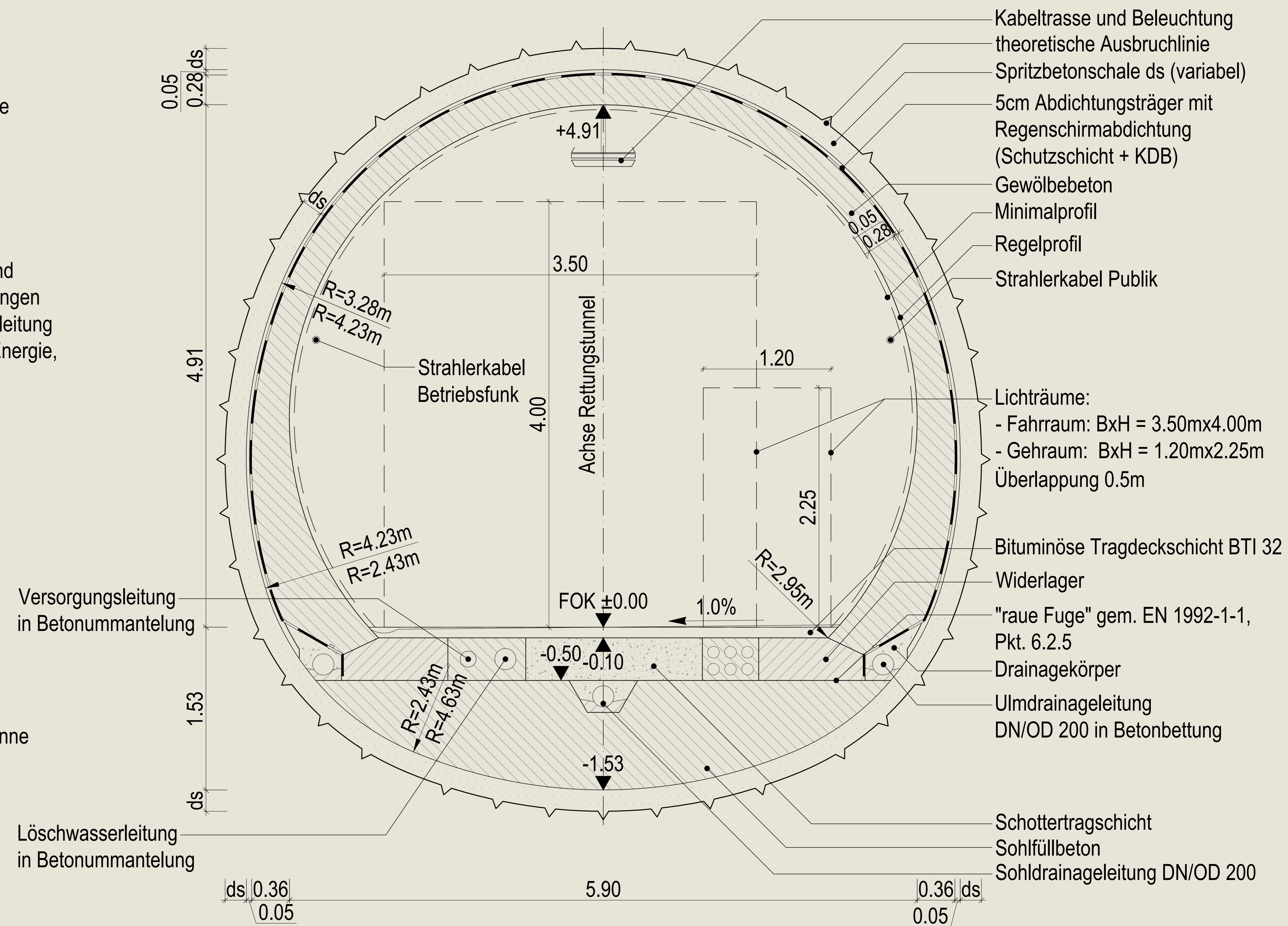
Rettungstunnel Angath mit Innenschale
