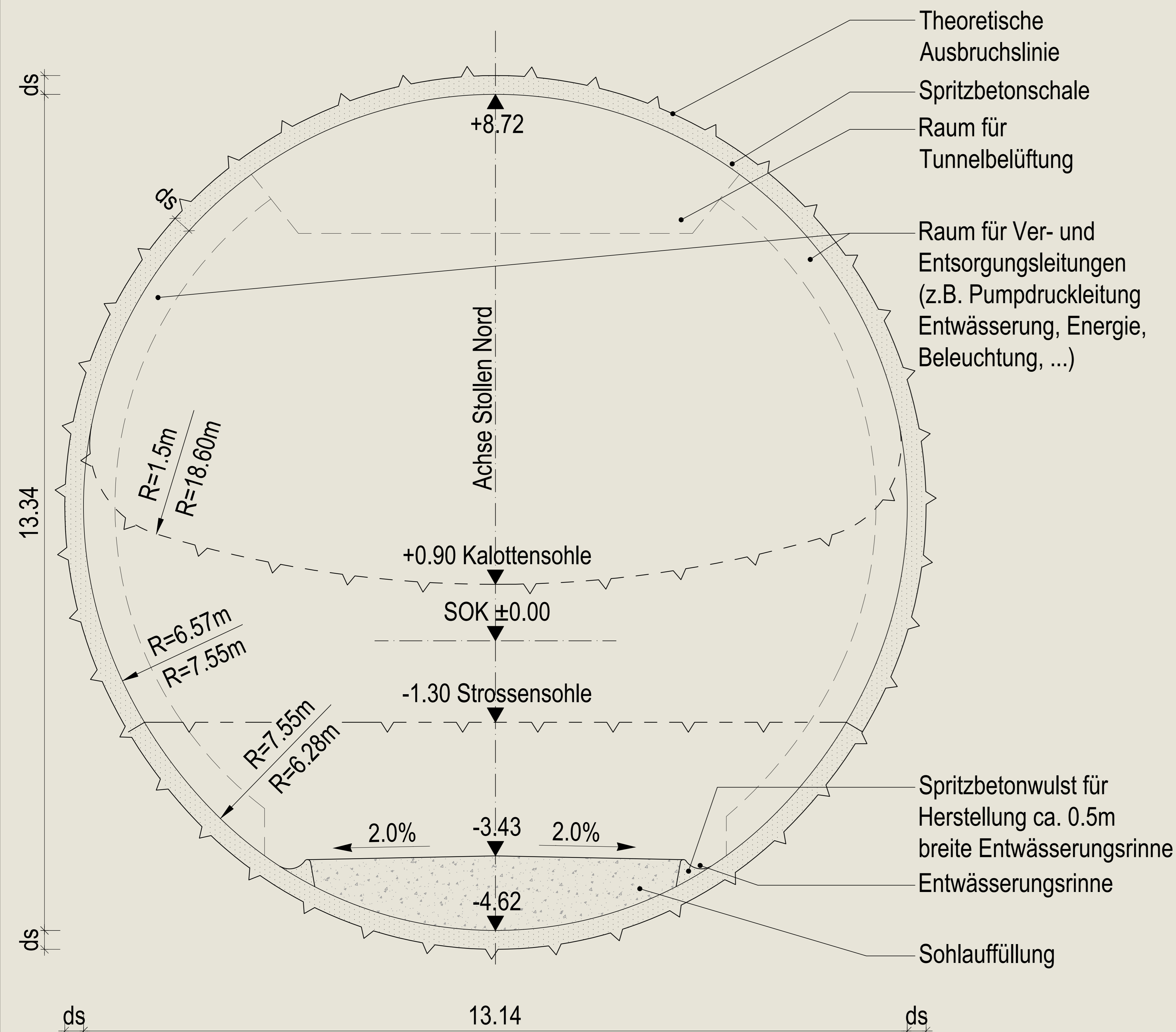
Stollen NORD (Angerbergtunnel) ohne Innenschale
