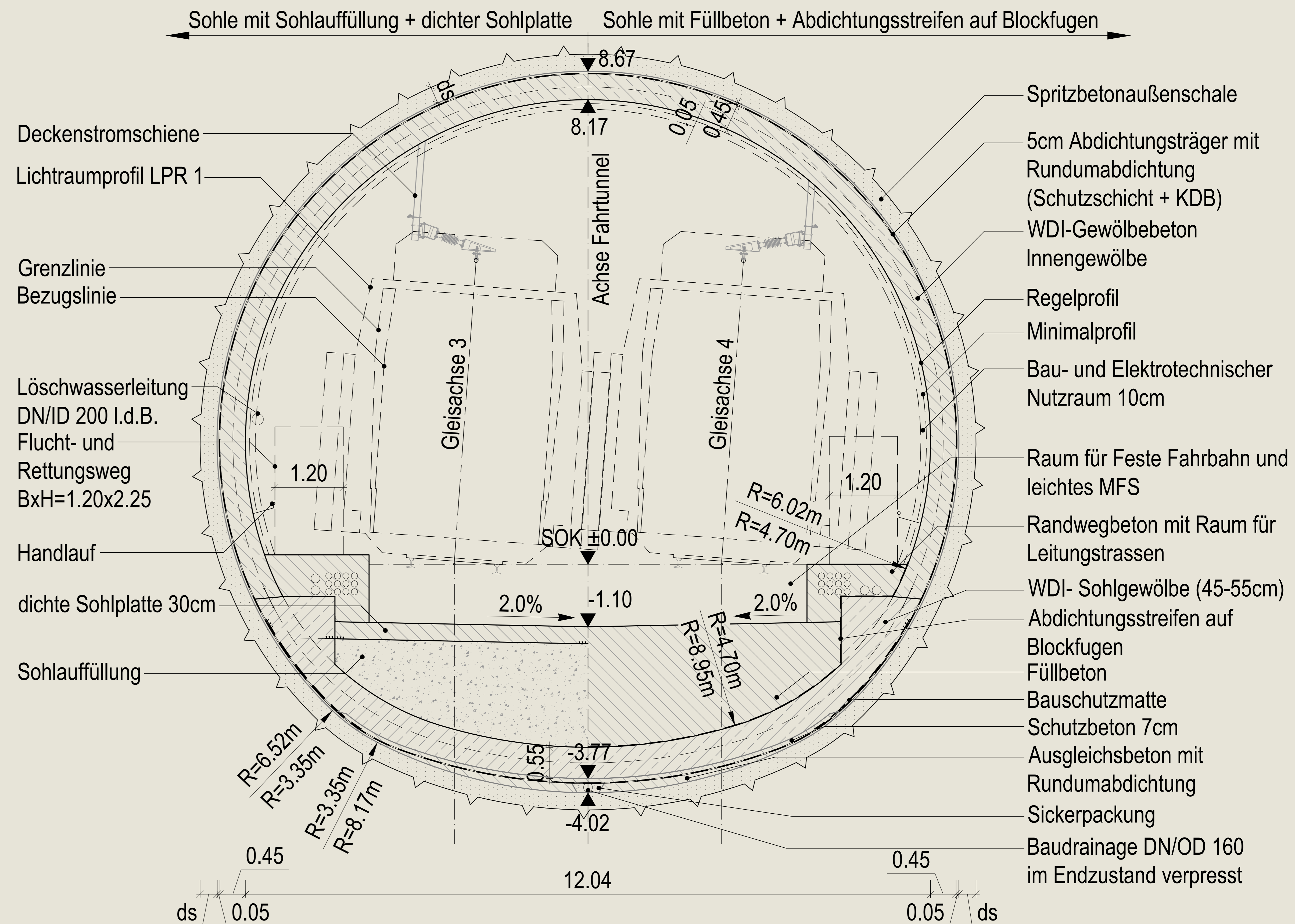
Angerbergtunnel mit Innenschale
