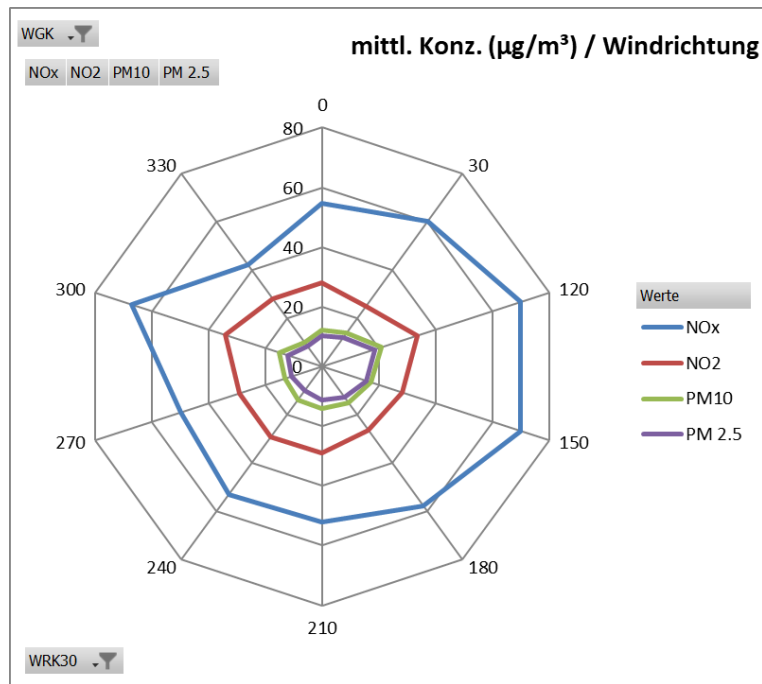
Abbildung 11 Windrichtungsabhängigkeit der Immissionsbelastung im Monat Dezember 2023 (es sind nur Datensätze mit Windgeschwindigkeiten > 0,5 m/s in der Darstellung berücksichtigt)
