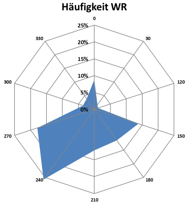
Abbildung 9 Windrichtungsverteilung im Monat Dezember 2023 (nur HMW mit Windgeschwindigkeiten > 0,5 m/s)
