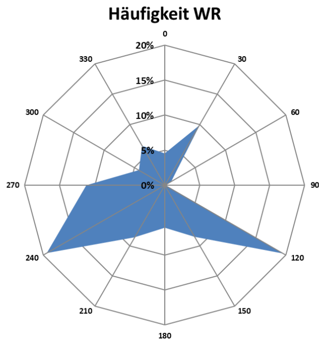
Abbildung 9 Windrichtungsverteilung im Monat Juli 2023 (nur HMW mit Windgeschwindigkeiten > 0,5 m/s)
