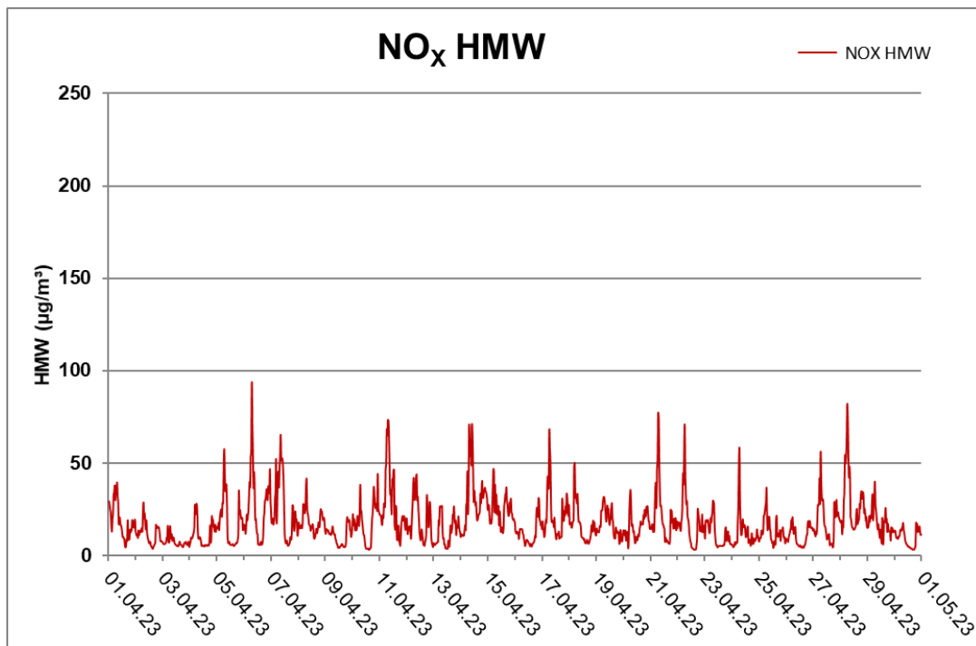
Abbildung 3 Zeitlicher Verlauf der NO x Halbstundenmittelwerte der Beweissicherungsmessstelle Angath
