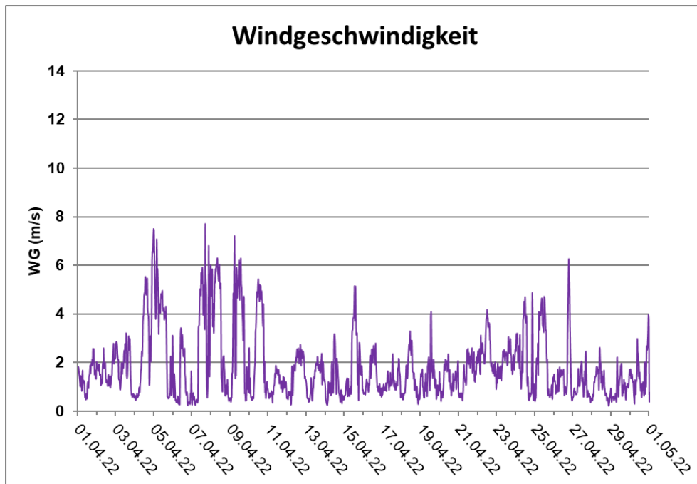
Abbildung 10 Zeitlicher Verlauf der Windgeschwindigkeiten
