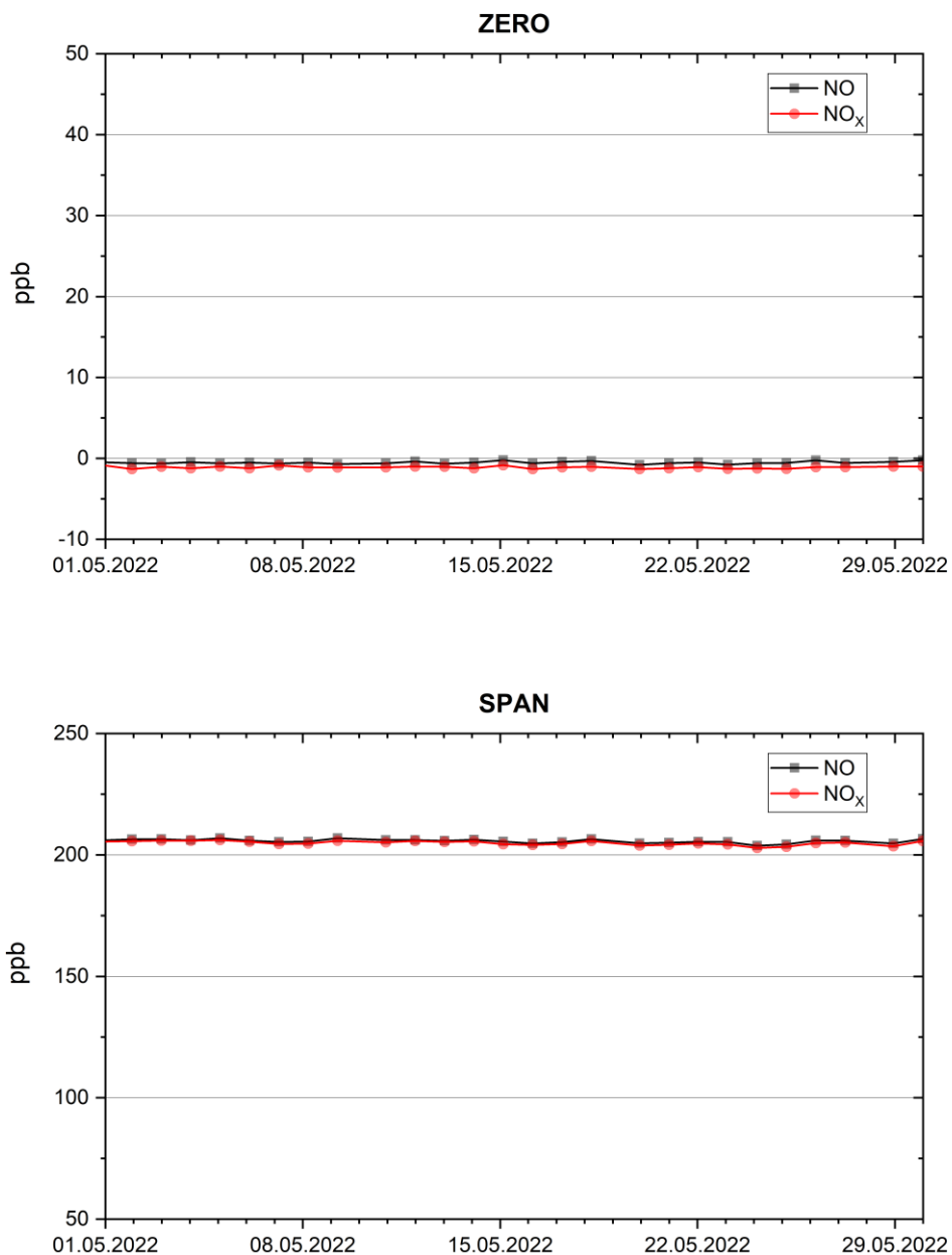
Abbildung 12: Verlauf vom Nullpunkt und Kalibrierwerten
