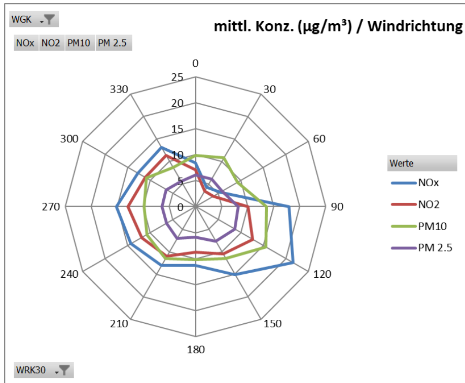
Abbildung 11 Windrichtungsabhängigkeit der Immissionsbelastung im Monat Mai 2022
